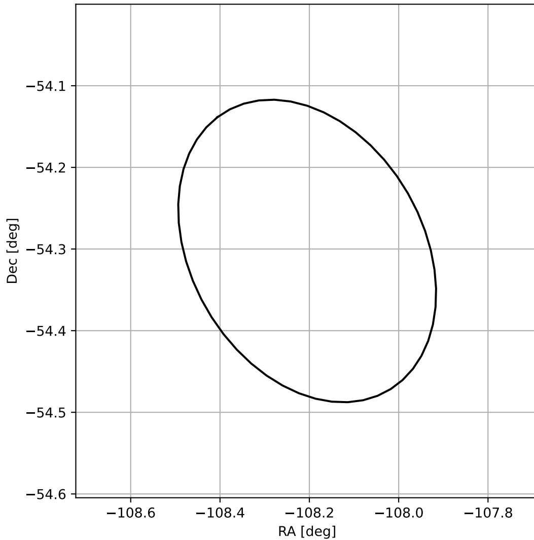
4FGL J1647.1-5418
