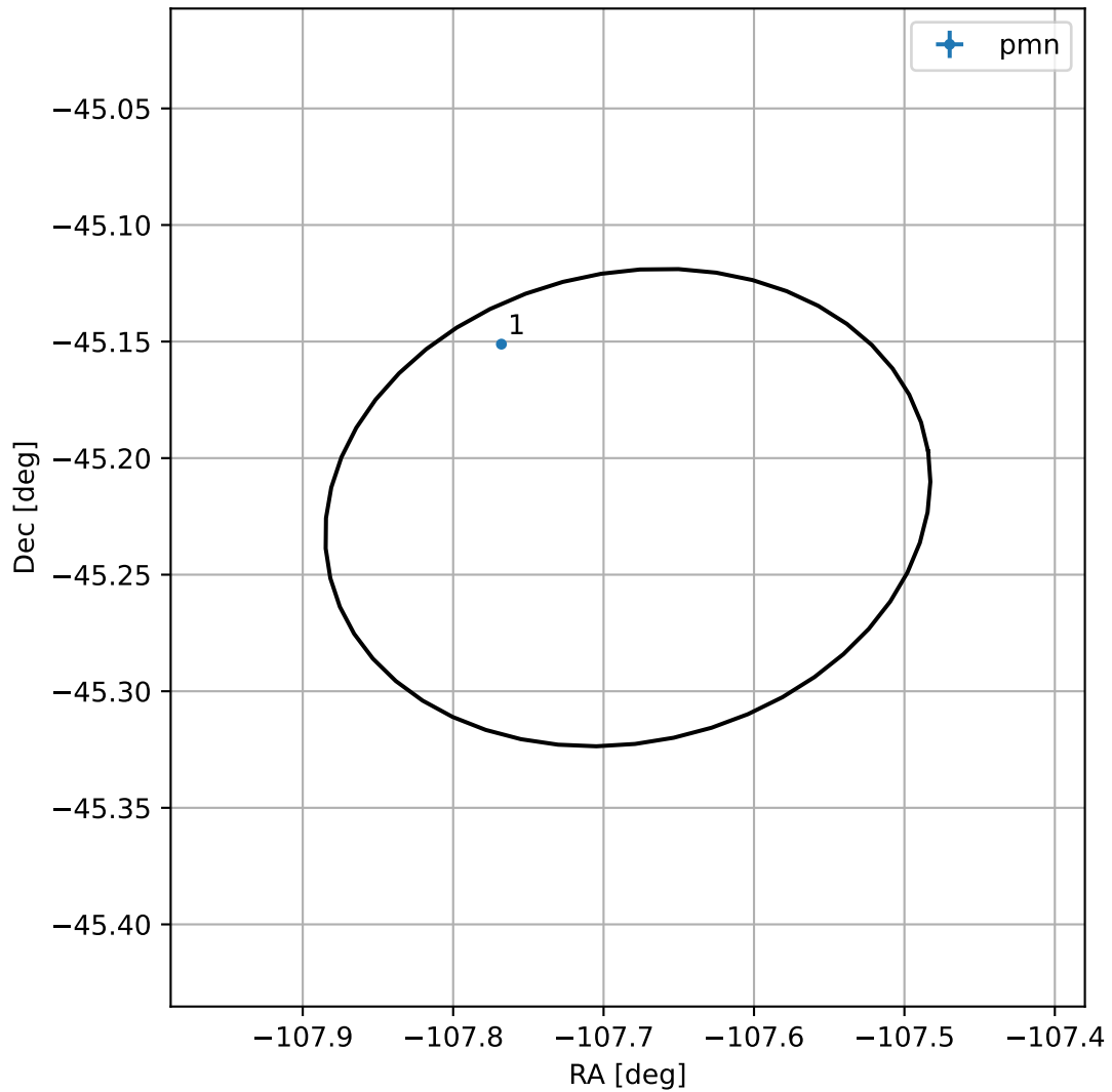
4FGL J1649.2-4513
