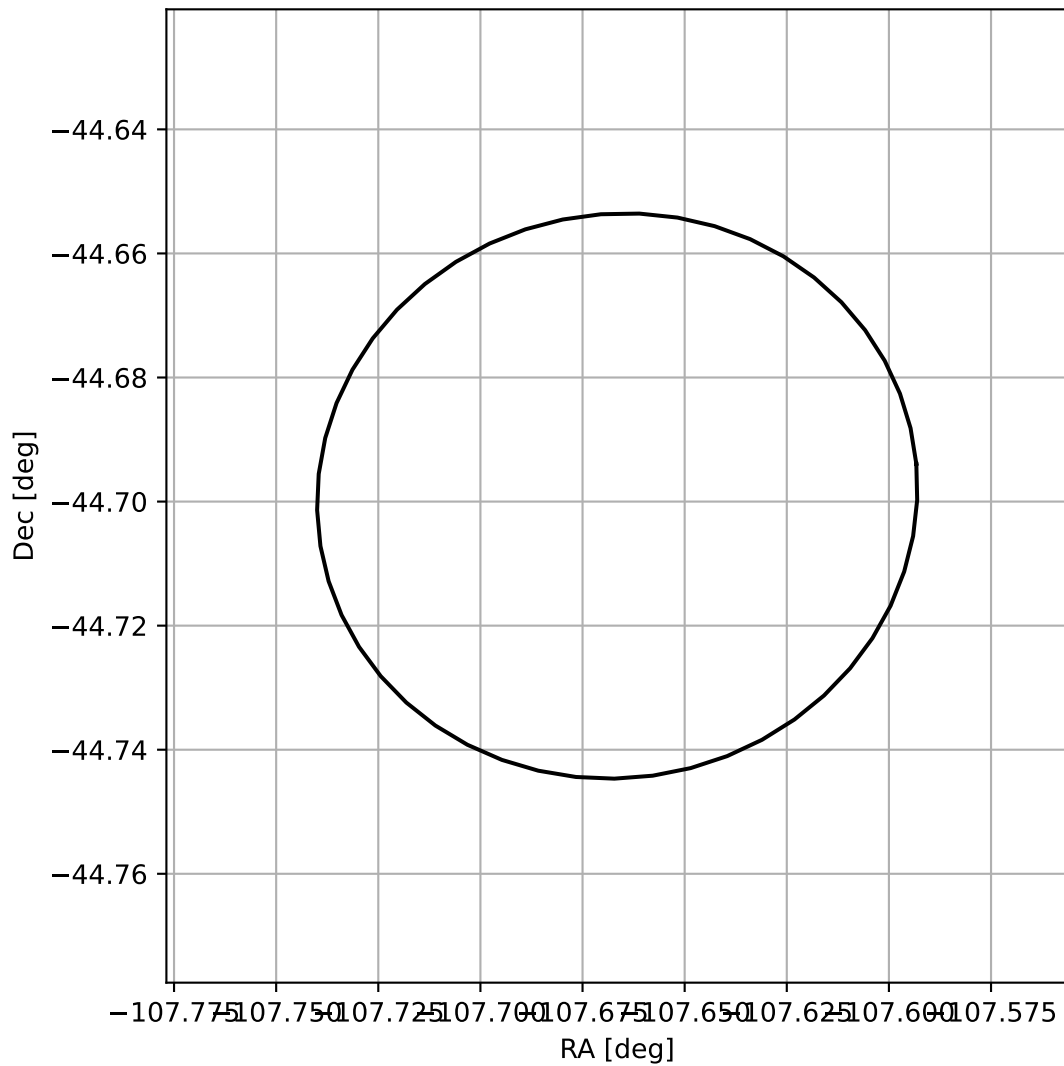
4FGL J1649.3-4441
