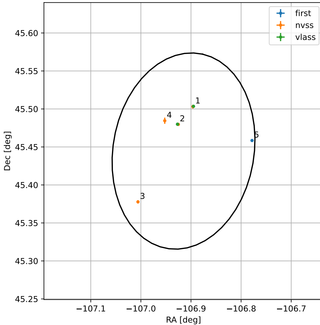
4FGL J1652.3+4526
