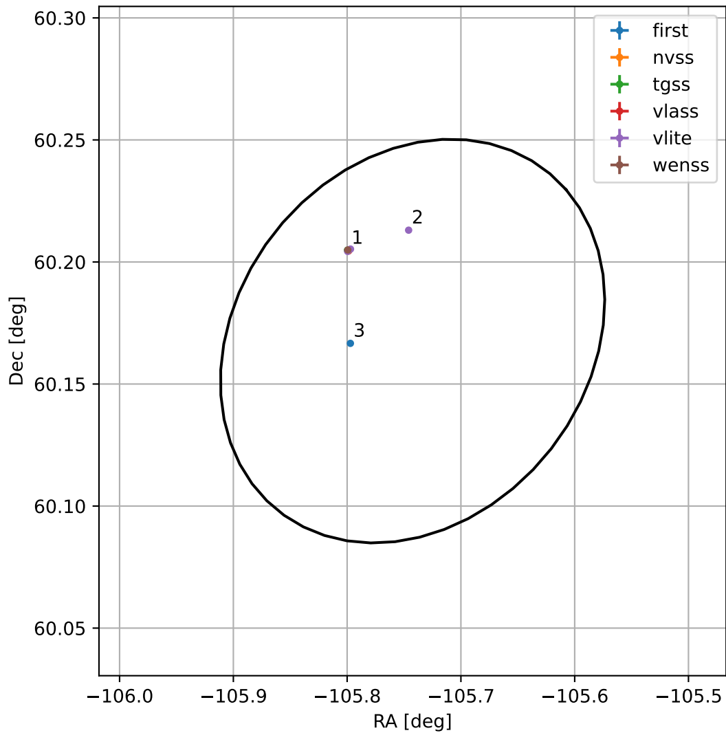
4FGL J1657.0+6010
