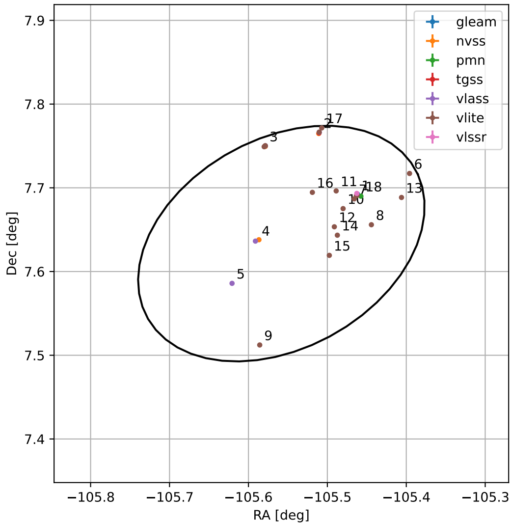
4FGL J1657.7+0738
