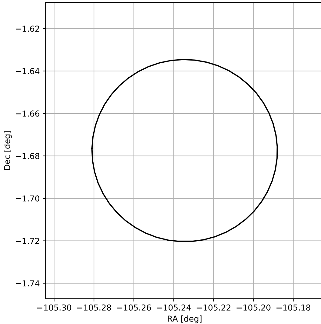
4FGL J1659.0-0140
