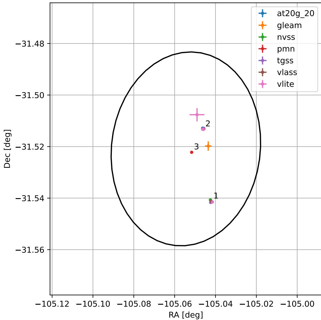
4FGL J1659.7-3131
