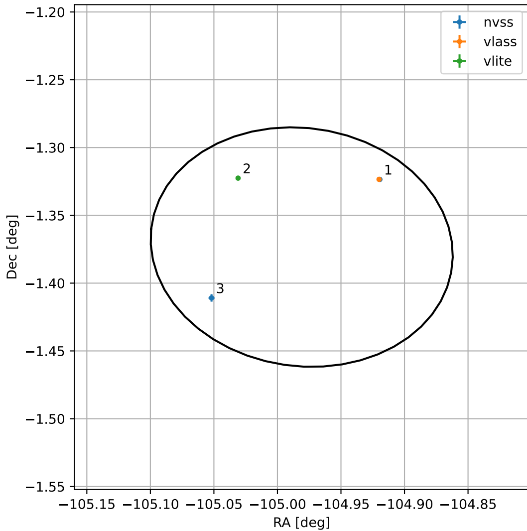
4FGL J1700.0-0122
