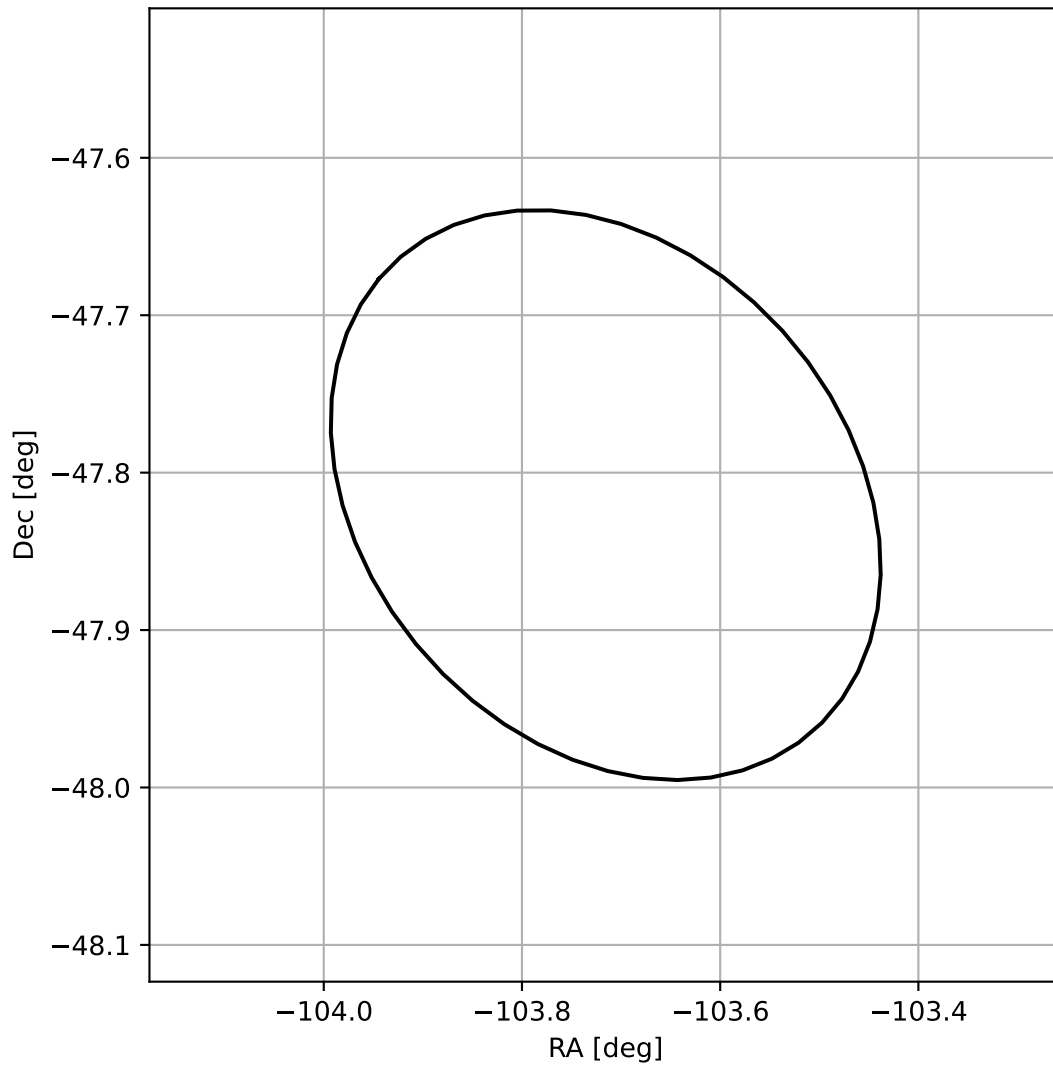
4FGL J1705.1-4748
