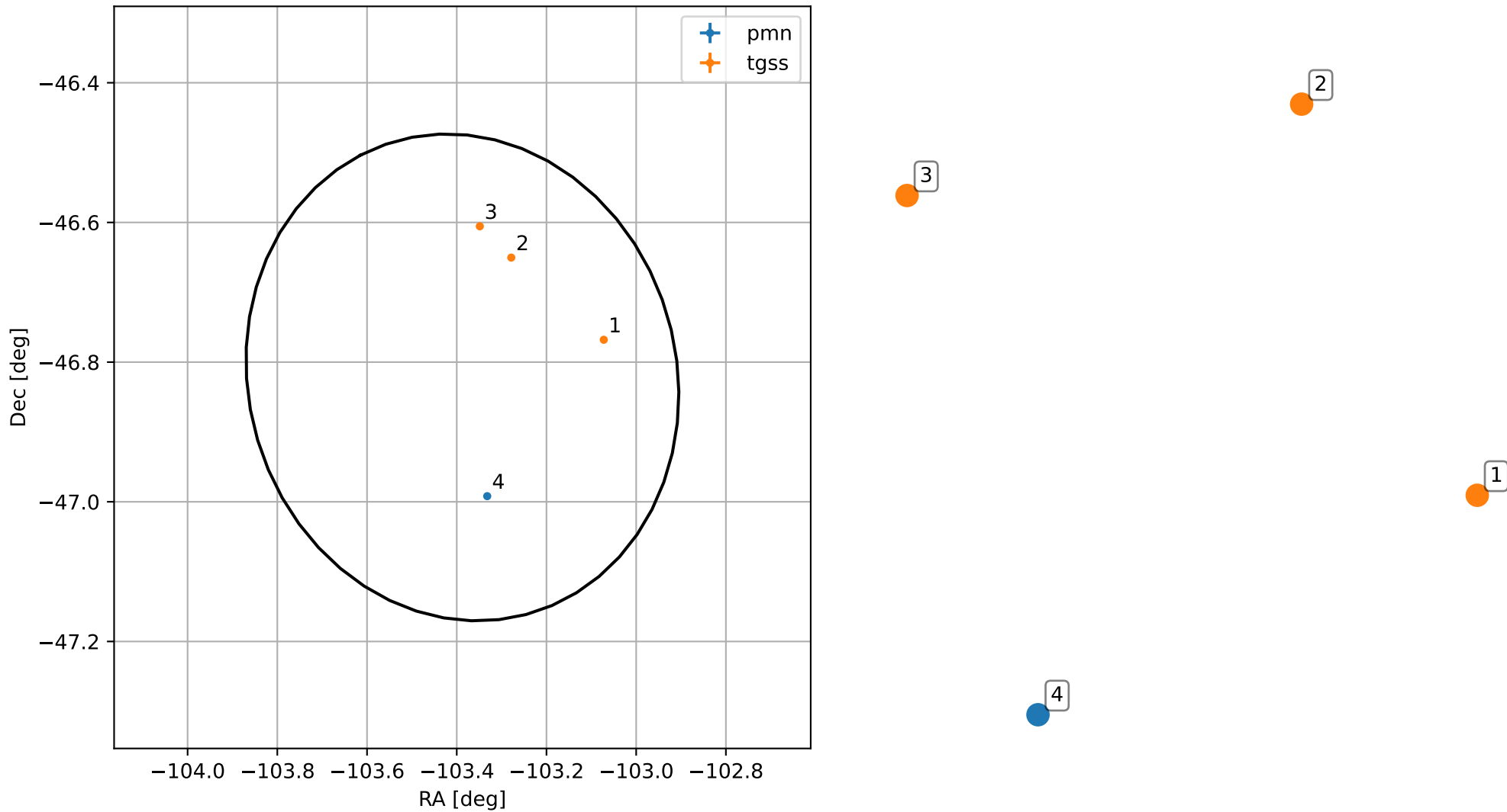
4FGL J1706.4-4649
