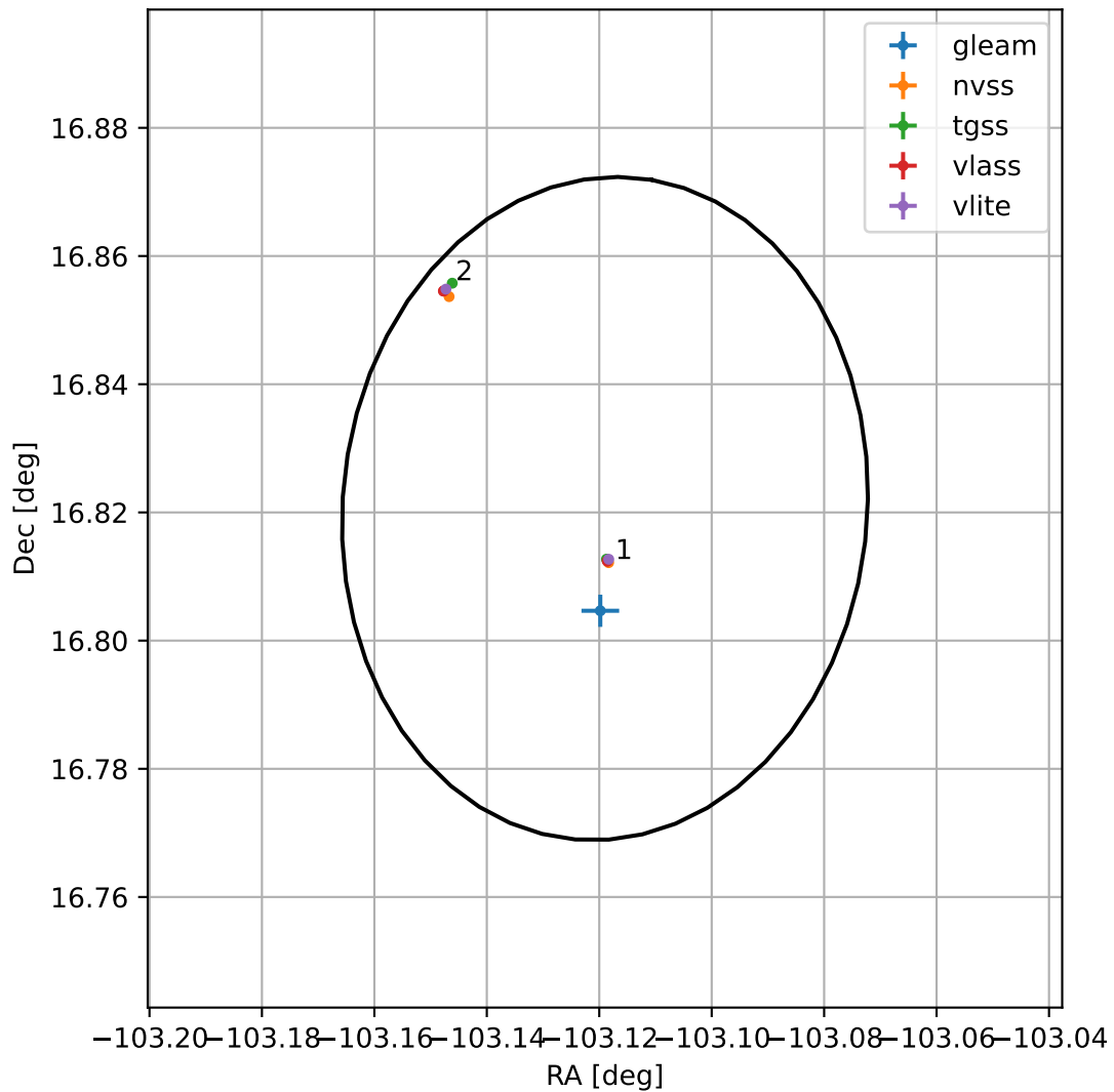
4FGL J1707.5+1649
