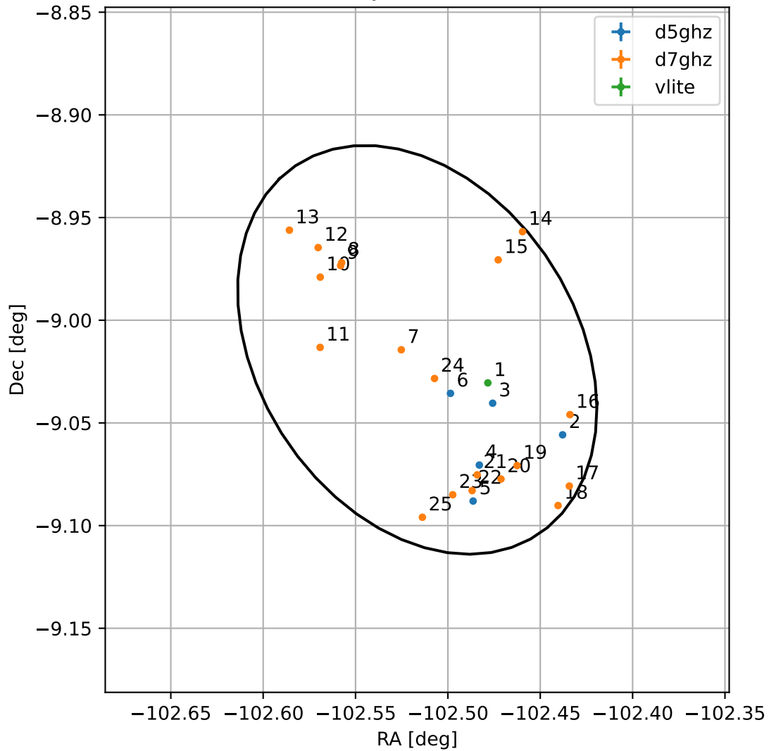
4FGL J1709.9-0900
