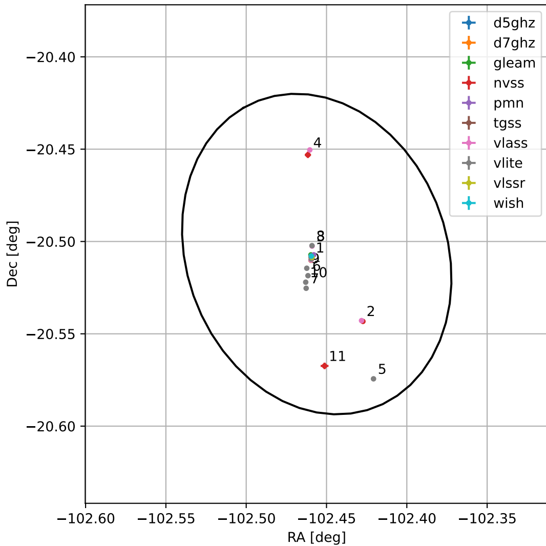
4FGL J1710.1-2030
