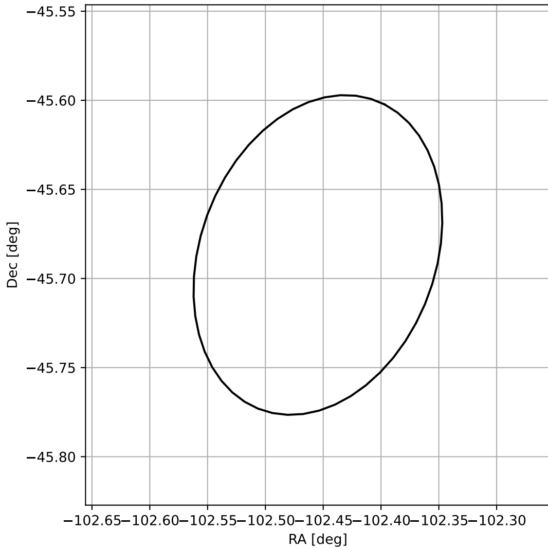
4FGL J1710.1-4541
