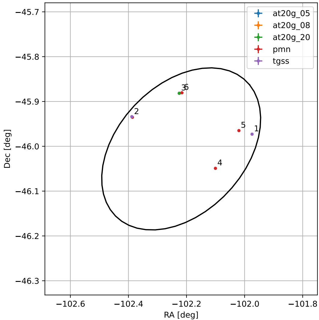
4FGL J1711.1-4600
