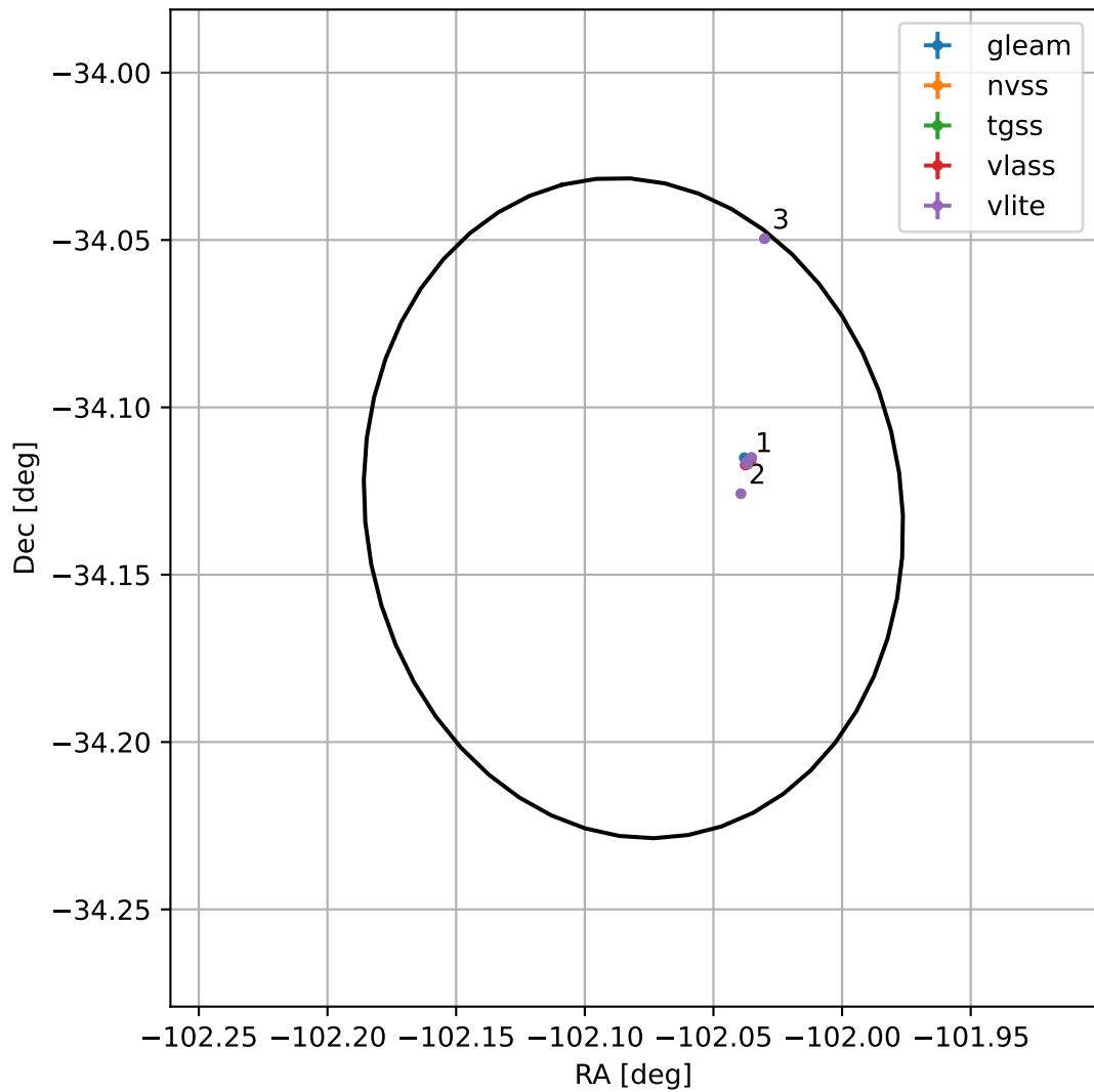
4FGL J1711.6-3407
