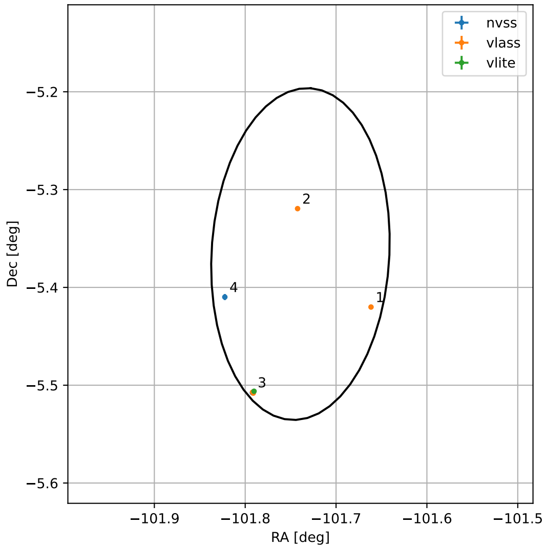
4FGL J1713.0-0521
