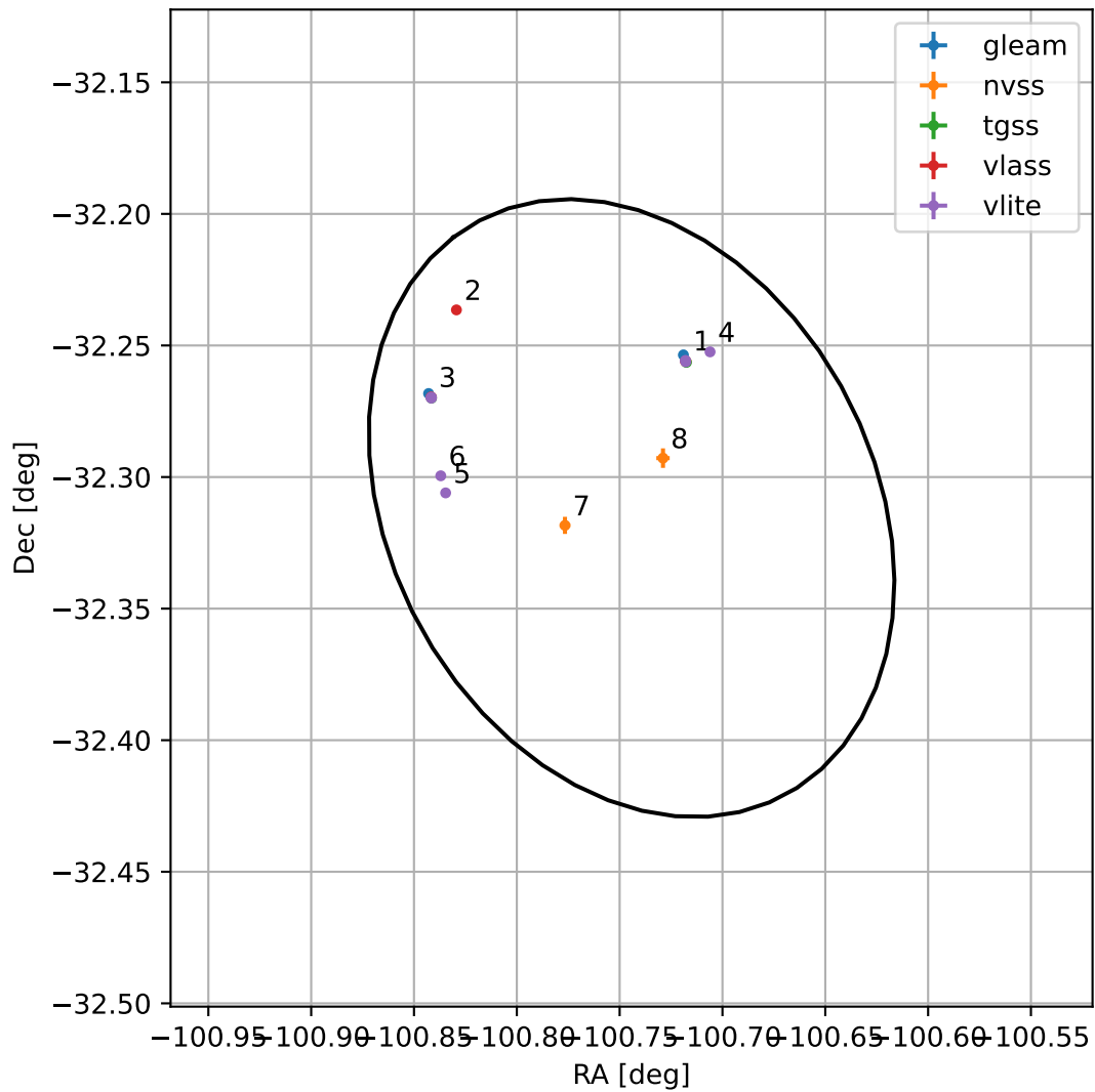
4FGL J1717.0-3218
