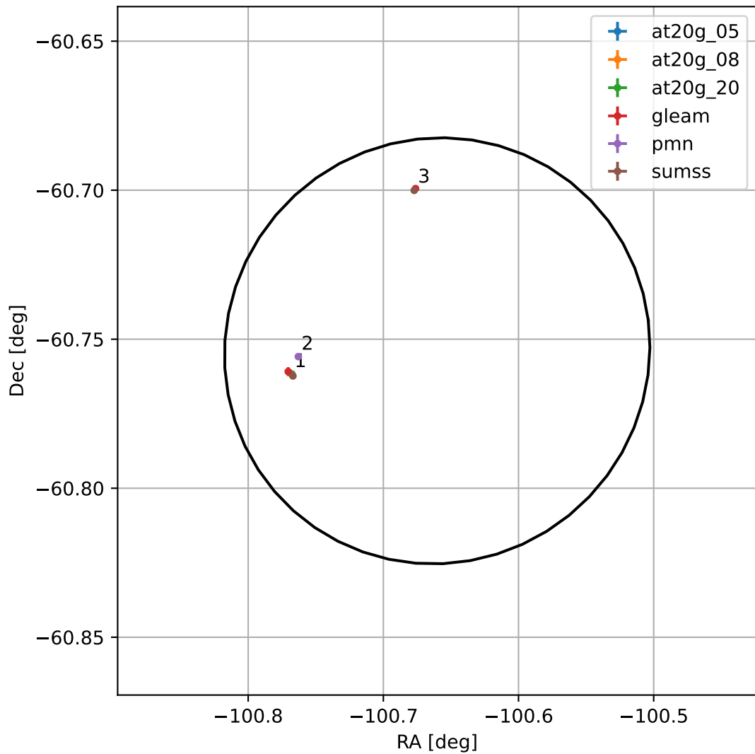
4FGL J1717.3-6045
