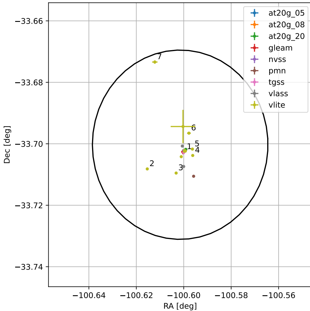
4FGL J1717.5-3342
