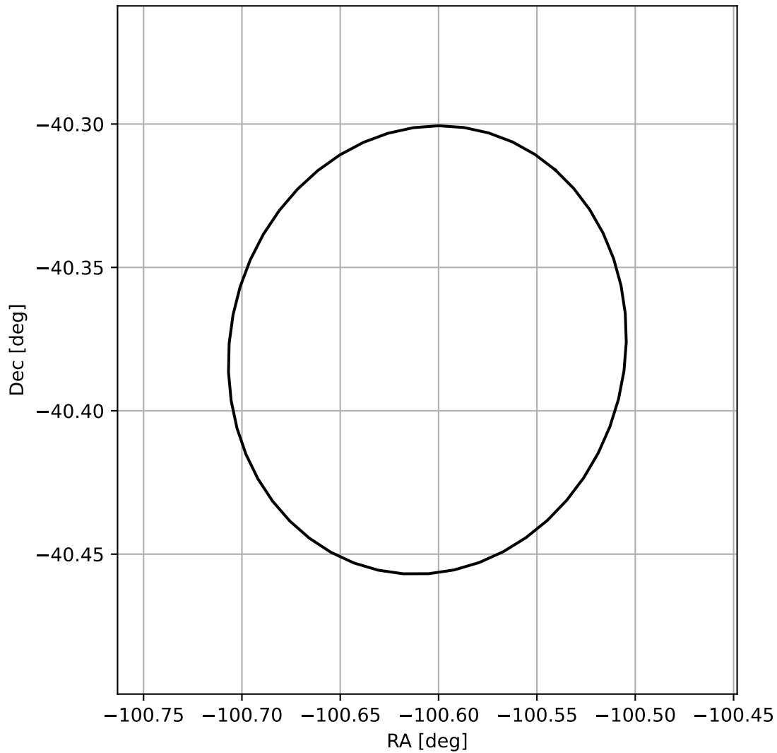
4FGL J1717.5-4022
