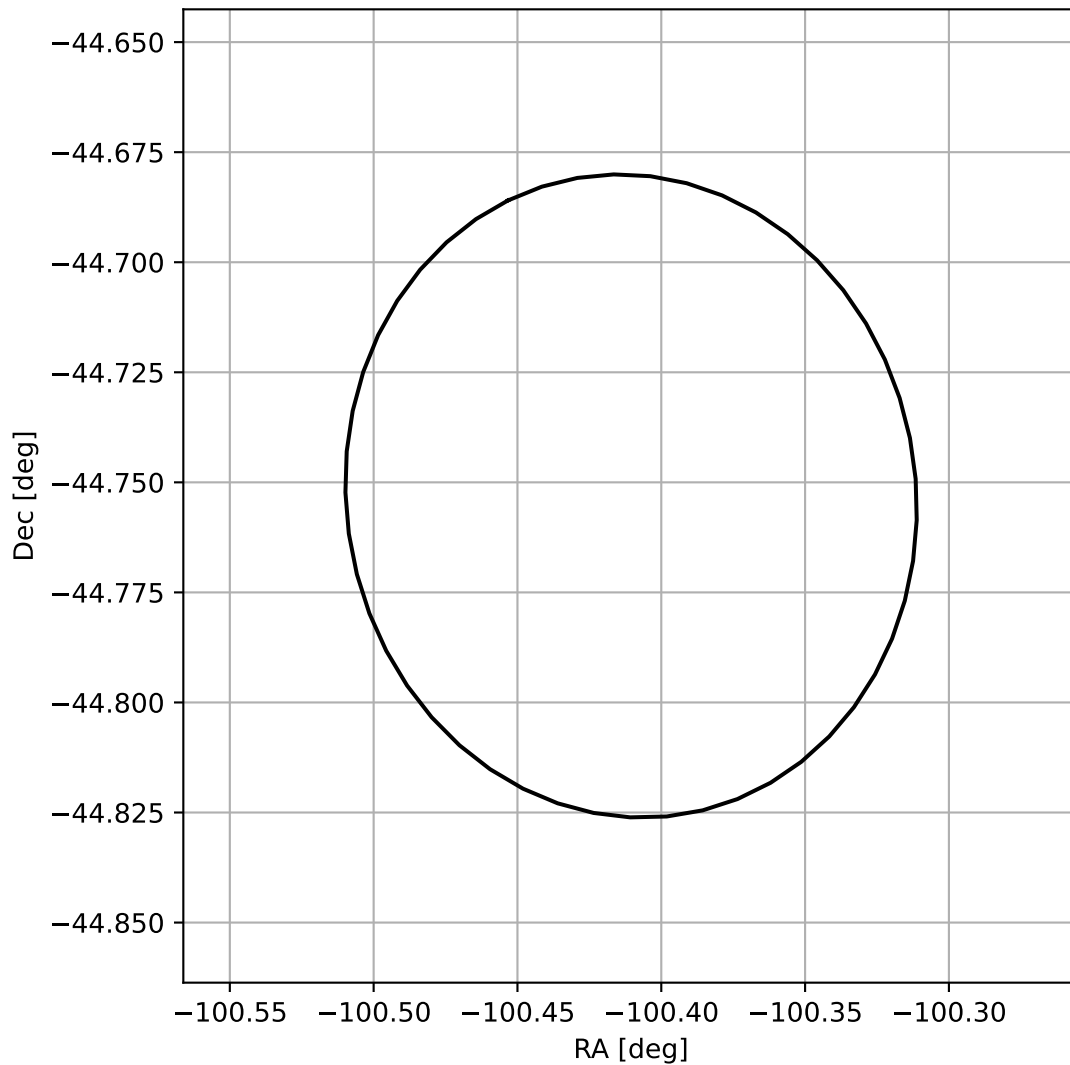
4FGL J1718.3-4445
