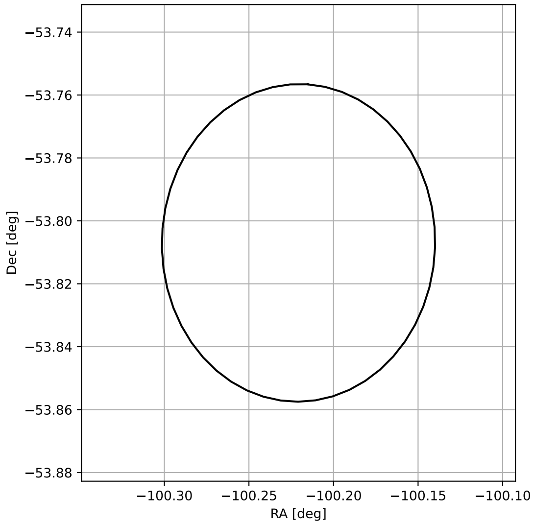
4FGL J1719.1-5348
