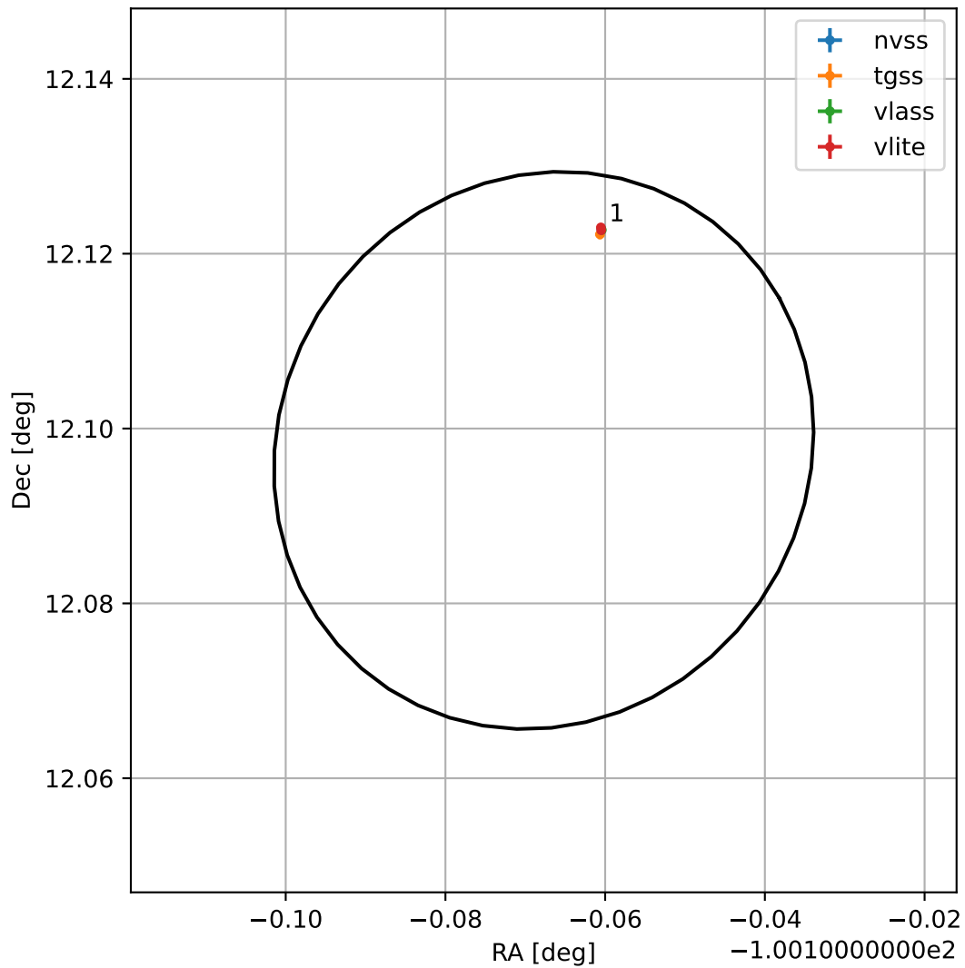
4FGL J1719.3+1205
