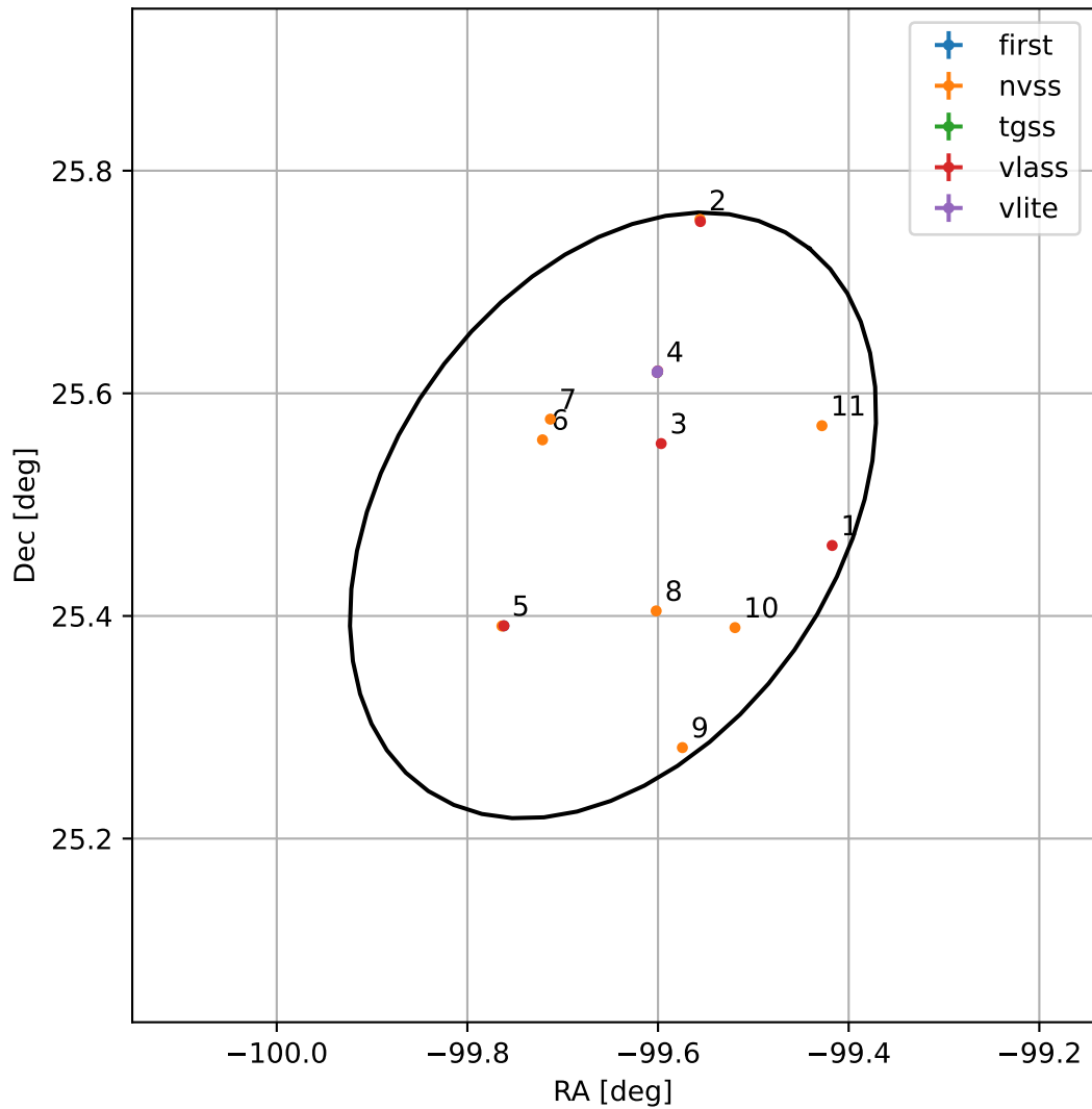
4FGL J1721.4+2529
