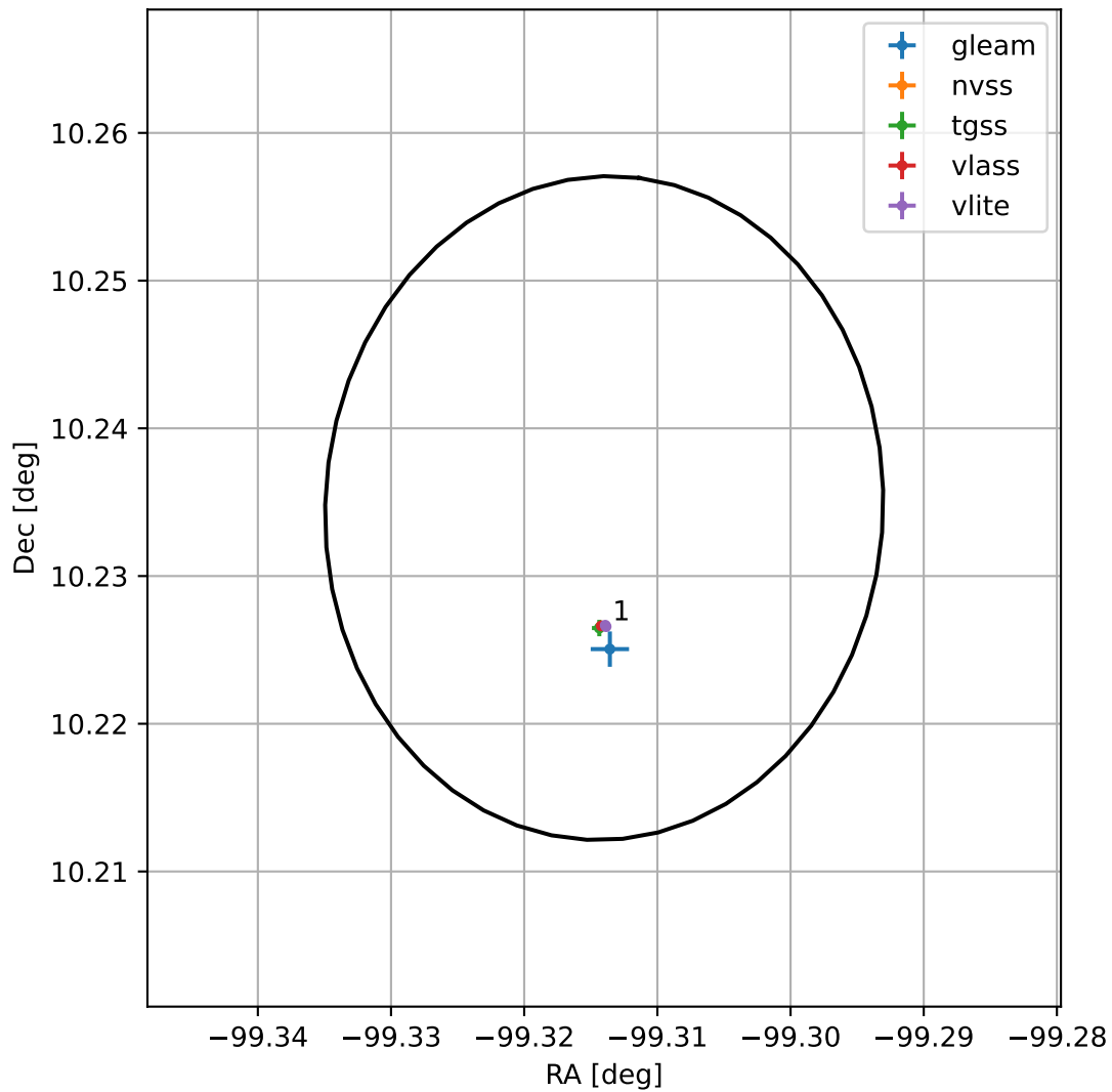
4FGL J1722.7+1014
