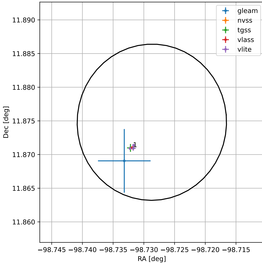
4FGL J1725.0+1152
