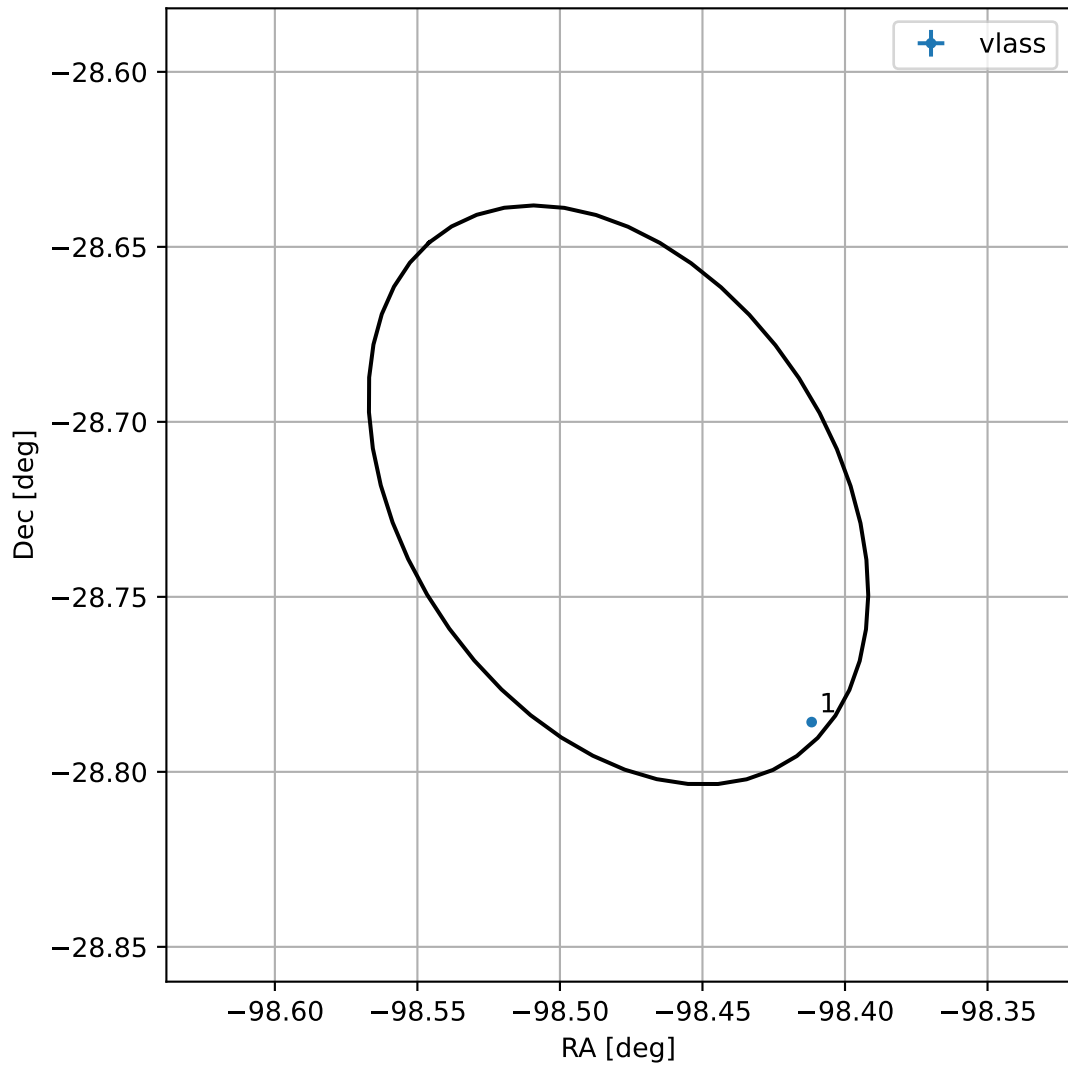
4FGL J1726.0-2843
