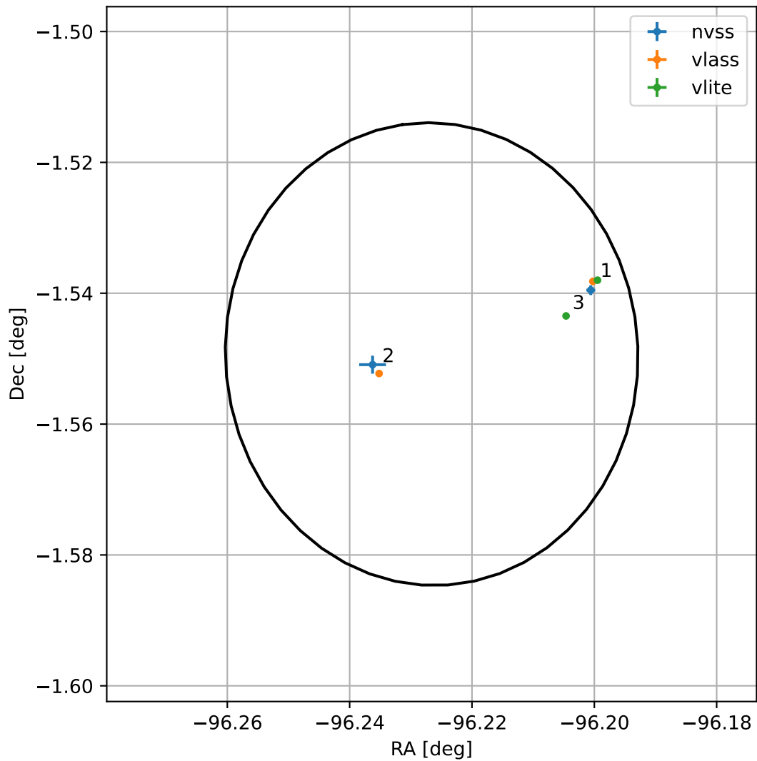
4FGL J1735.0-0132
