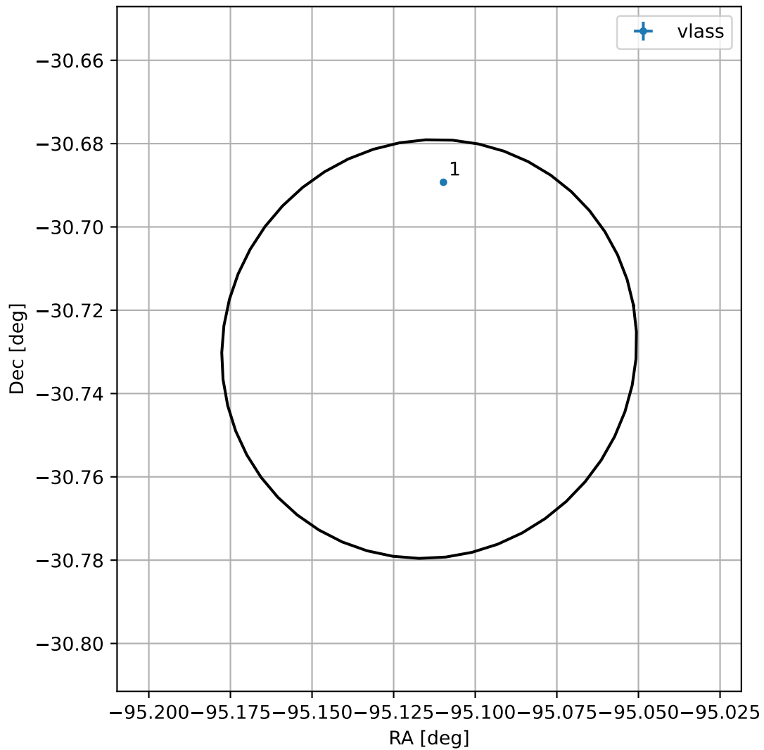
4FGL J1739.5-3043
