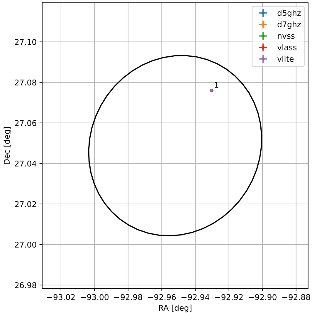
4FGL J1748.1+2702
