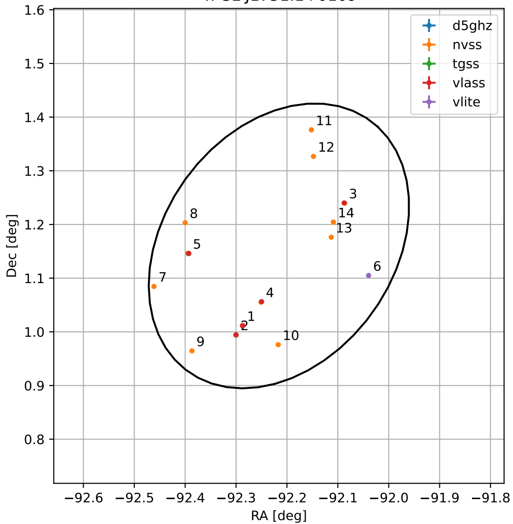
4FGL J1751.1+0109
