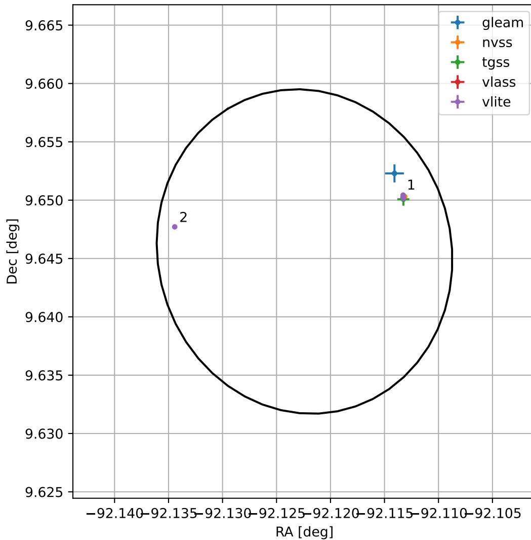
4FGL J1751.5+0938
