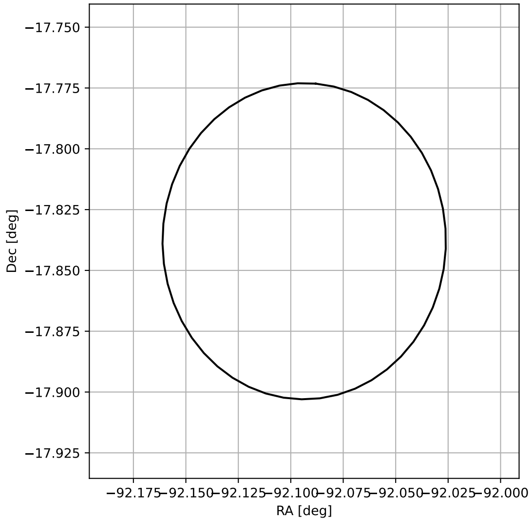
4FGL J1751.6-1750
