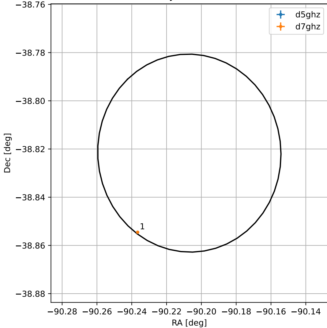
4FGL J1759.1-3849
