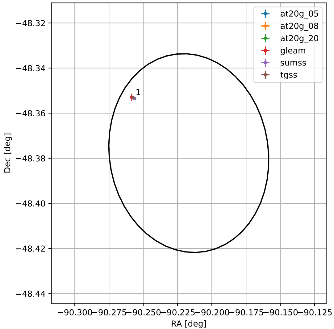
4FGL J1759.1-4822
