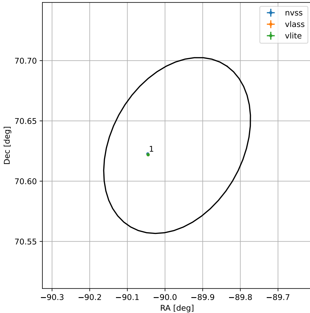
4FGL J1800.1+7037
