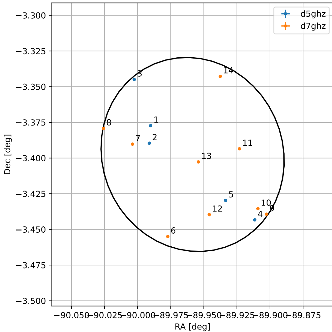
4FGL J1800.1-0323
