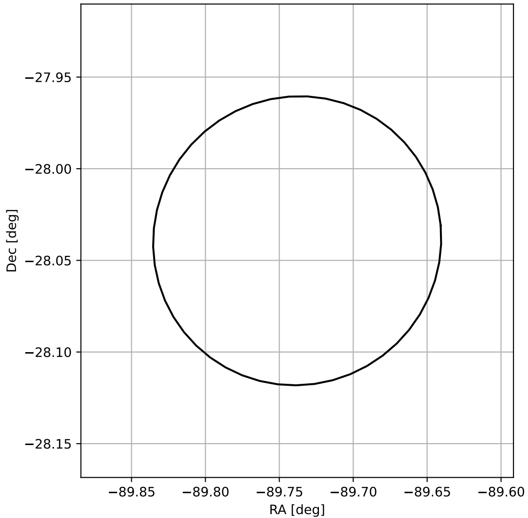
4FGL J1801.0-2802
