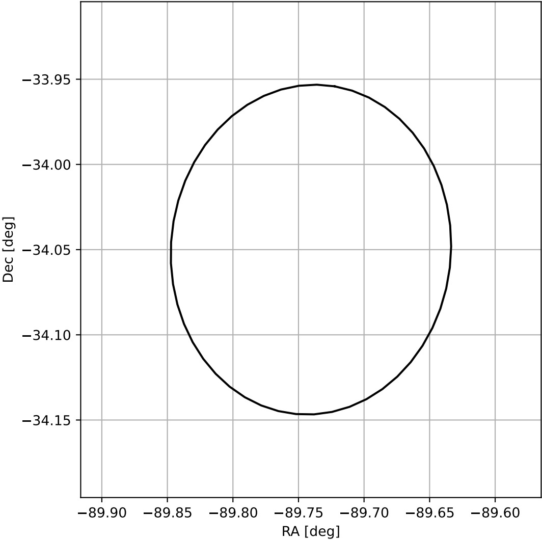
4FGL J1801.0-3402
