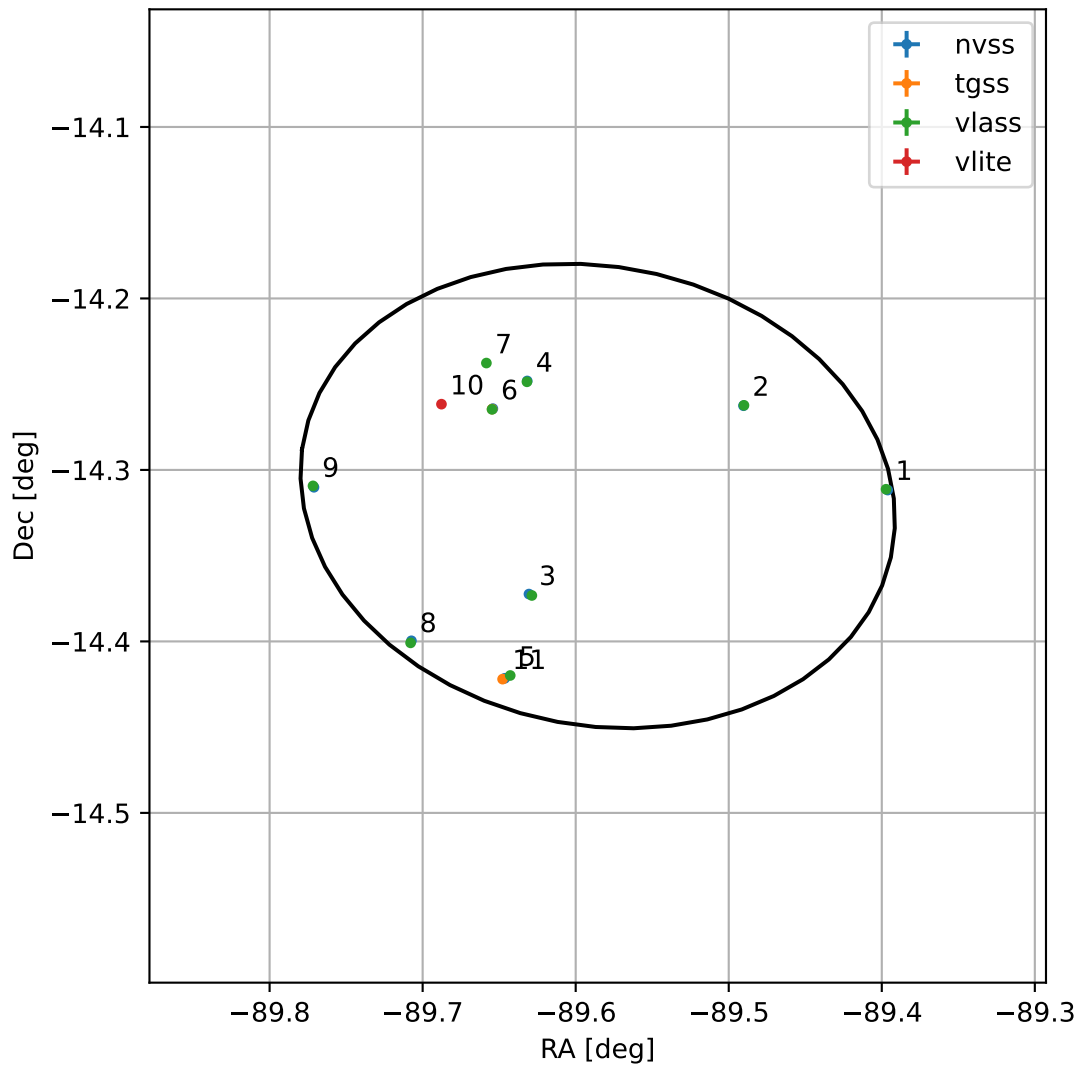
4FGL J1801.6-1418
