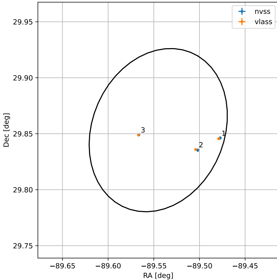
4FGL J1801.8+2951
