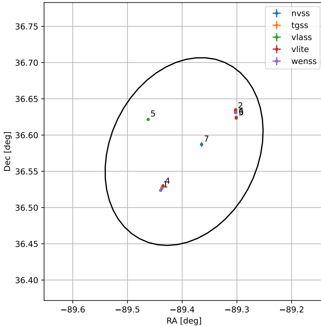
4FGL J1802.4+3634
