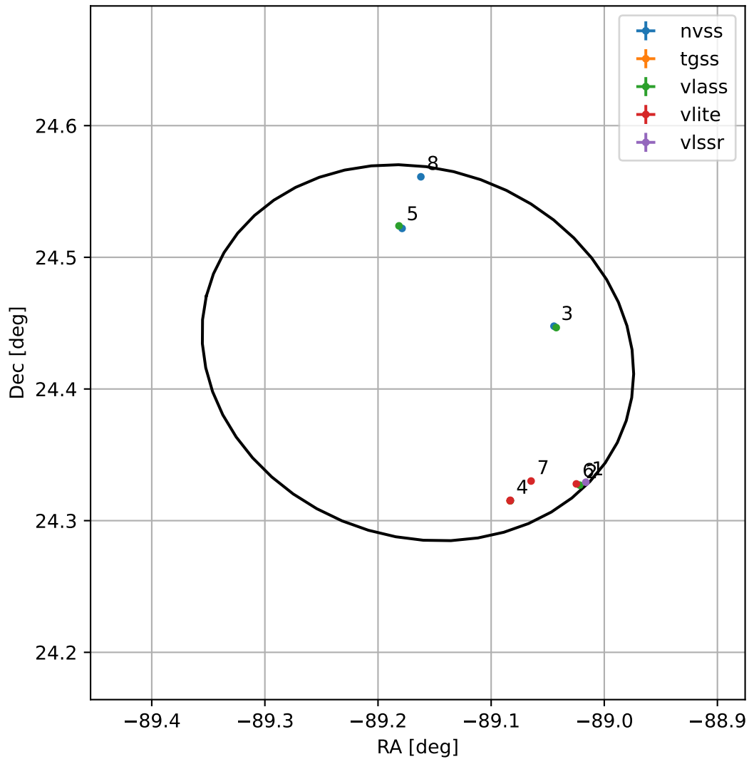
4FGL J1803.3+2425
