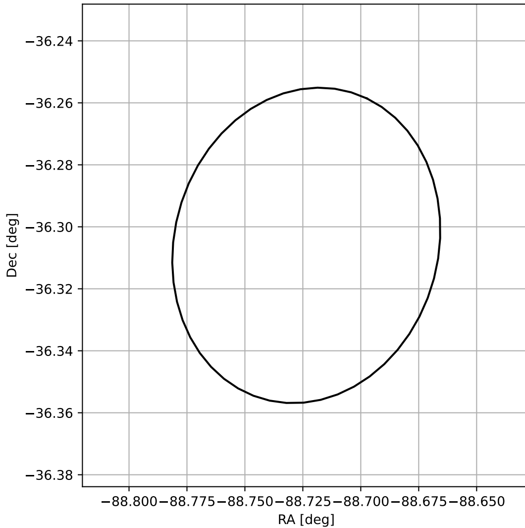
4FGL J1805.1-3618
