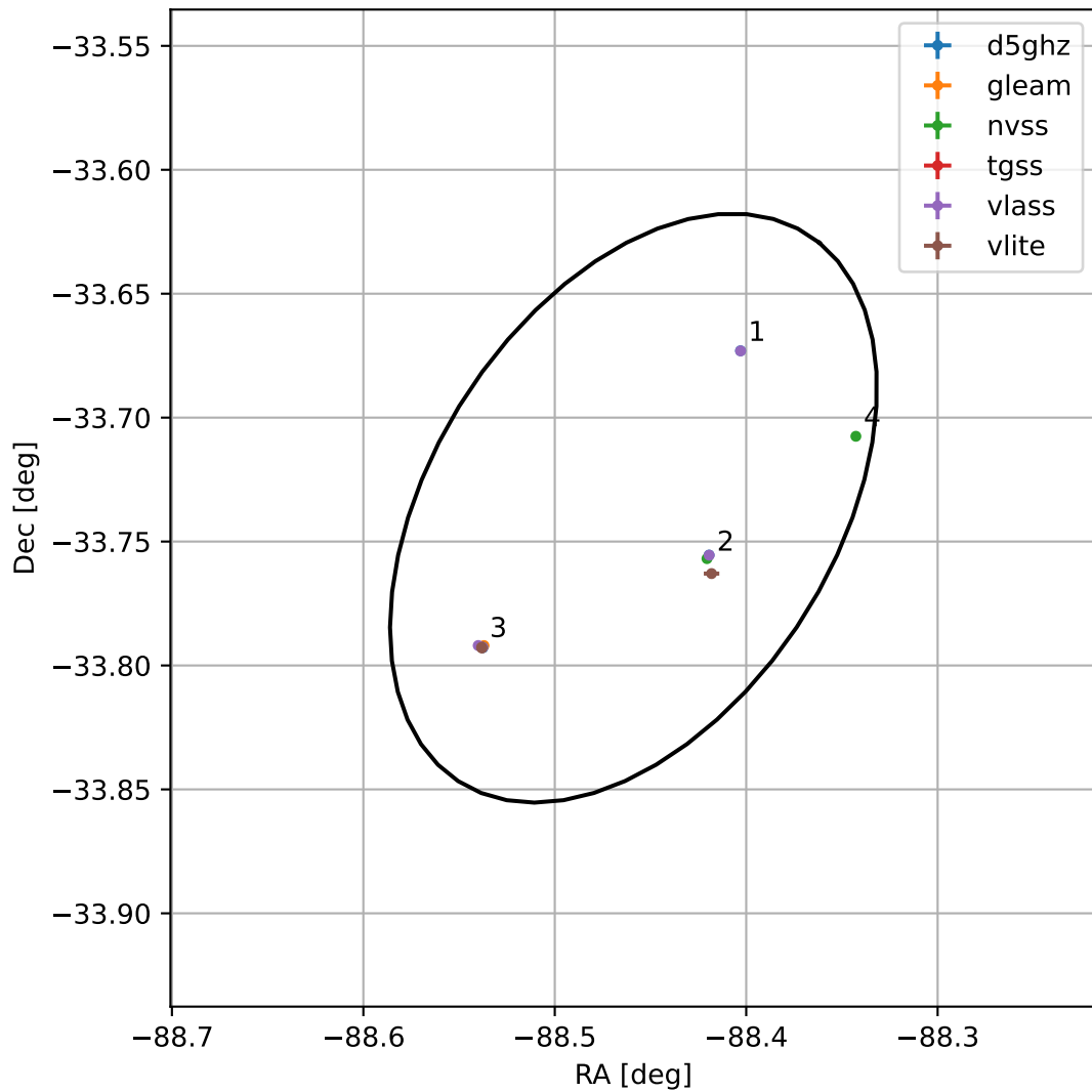
4FGL J1806.1-3344
