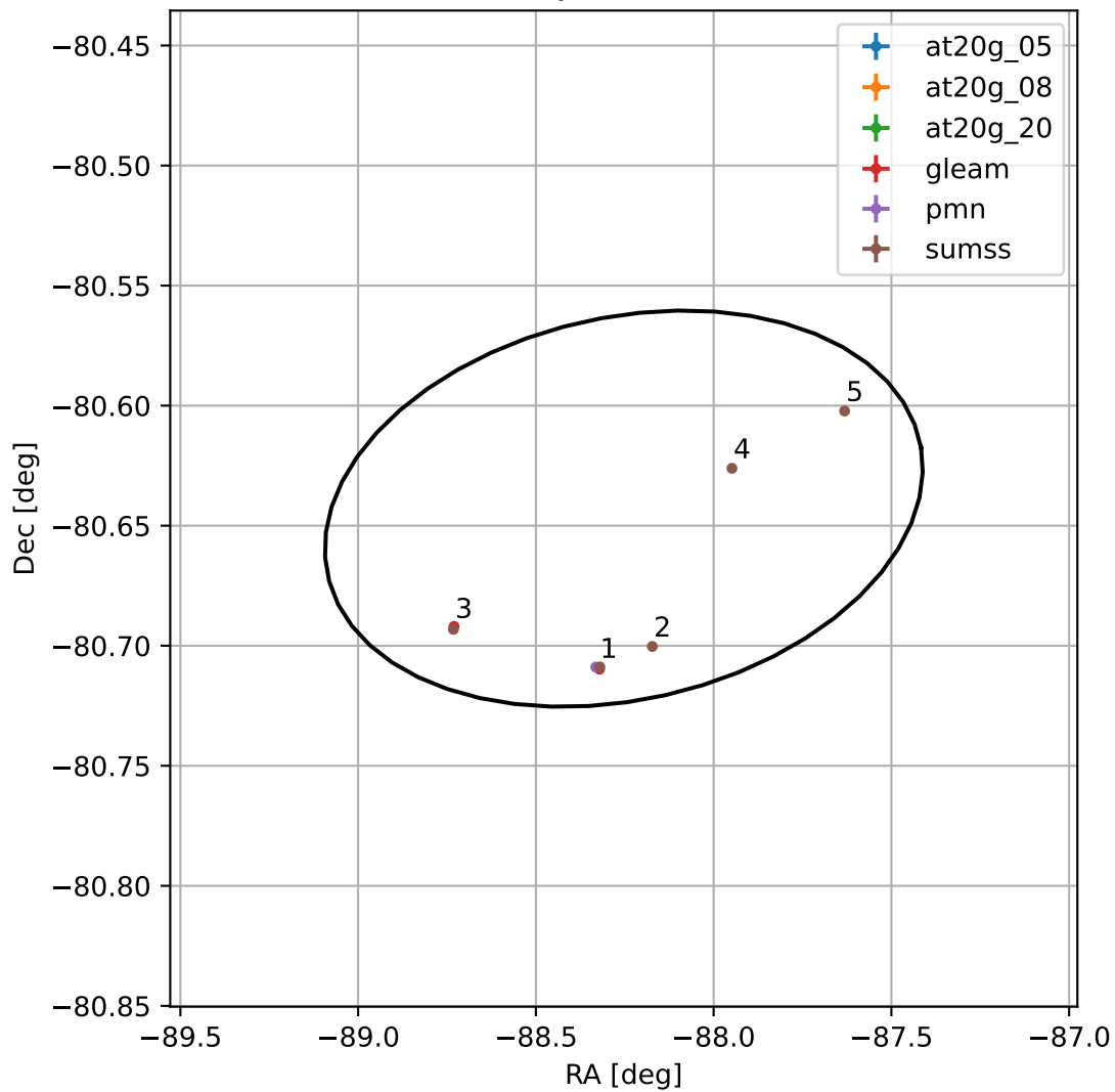
4FGL J1806.9-8038
