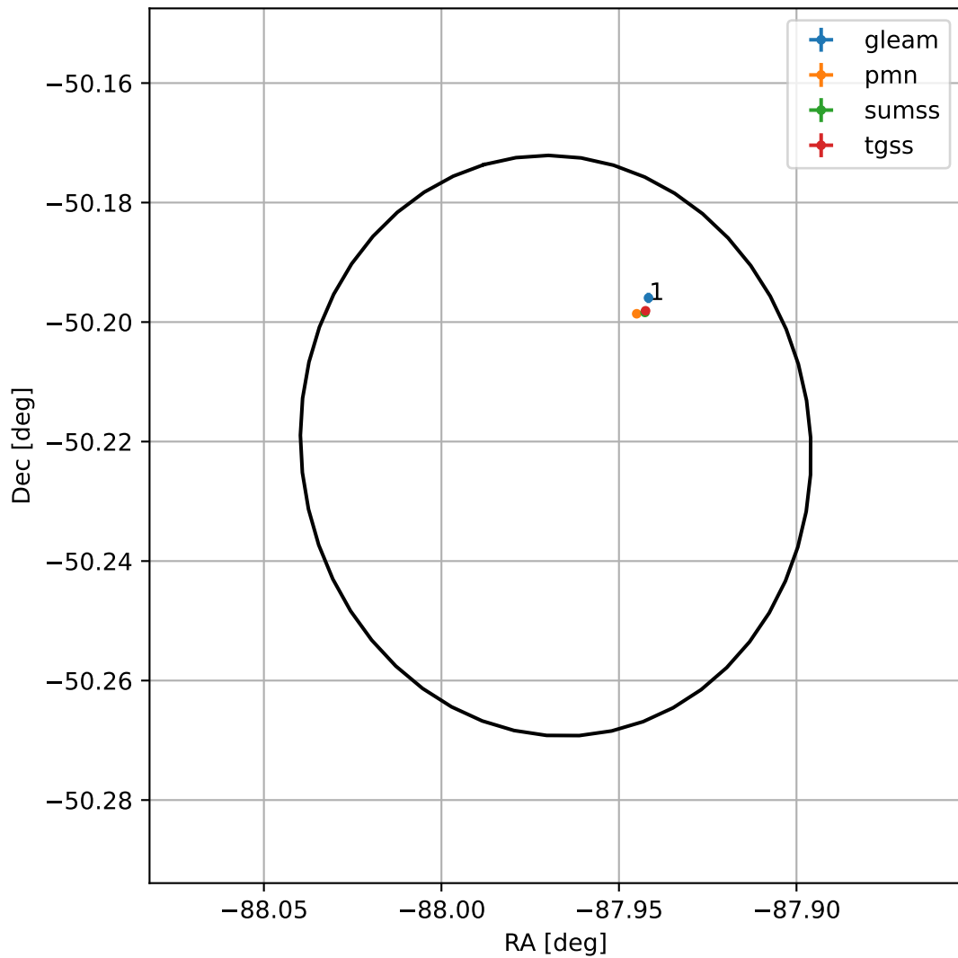
4FGL J1808.1-5013
