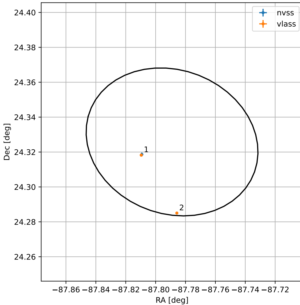
4FGL J1808.8+2419
